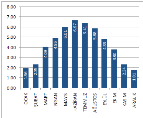
Şekil 46: GEPA Osmaniye ay bazlı günlük küresel radyasyon (güneş ışınması), 4 kWh/m 2
