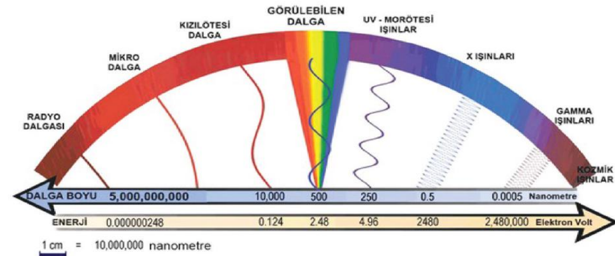
Şekil 27: Elektromanyetik spektrum
