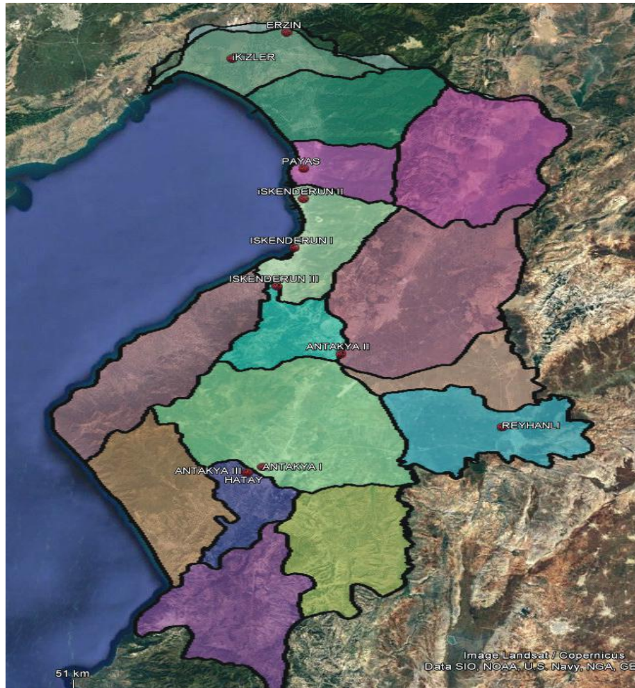
Şekil 68: Hatay TEİAŞ trafo merkezleri
