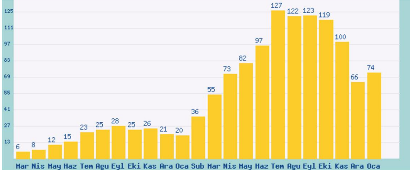
Şekil 6: 2017 yılı Ocak ayı ve öncesi 24 aylık dönemde güneş enerjisi ile gerçekleştirilen elektrik üretimi (Kaynak: TEİAŞ)
